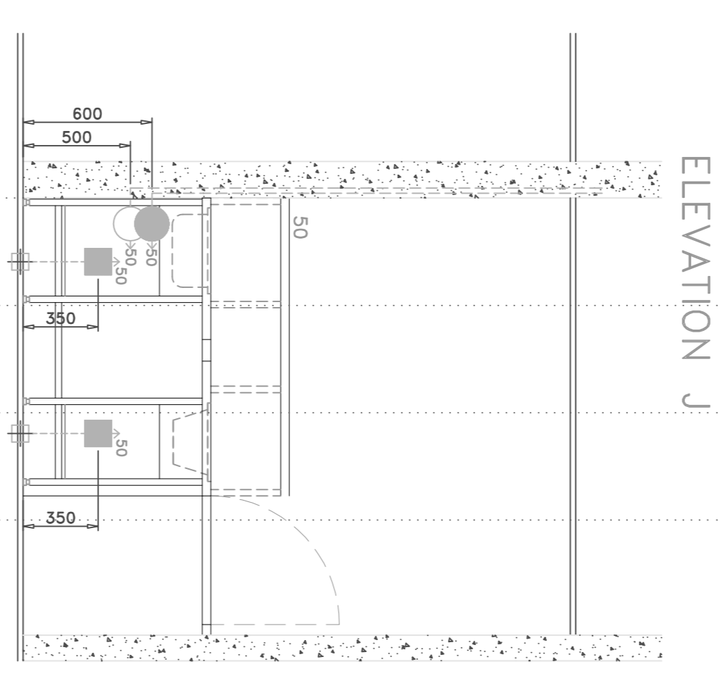
ELEVATION J
