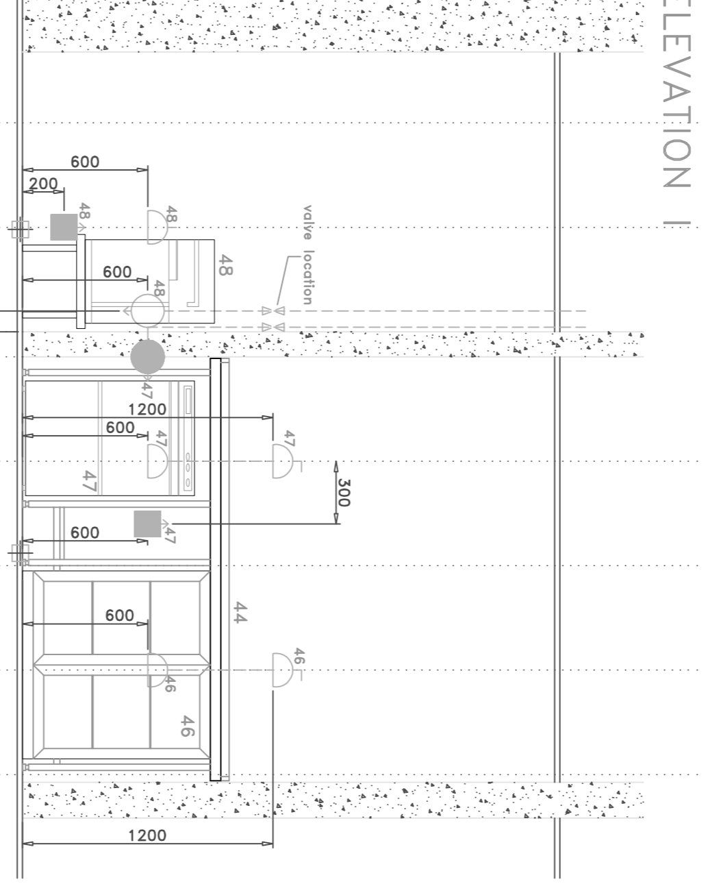
ELEVATION I
