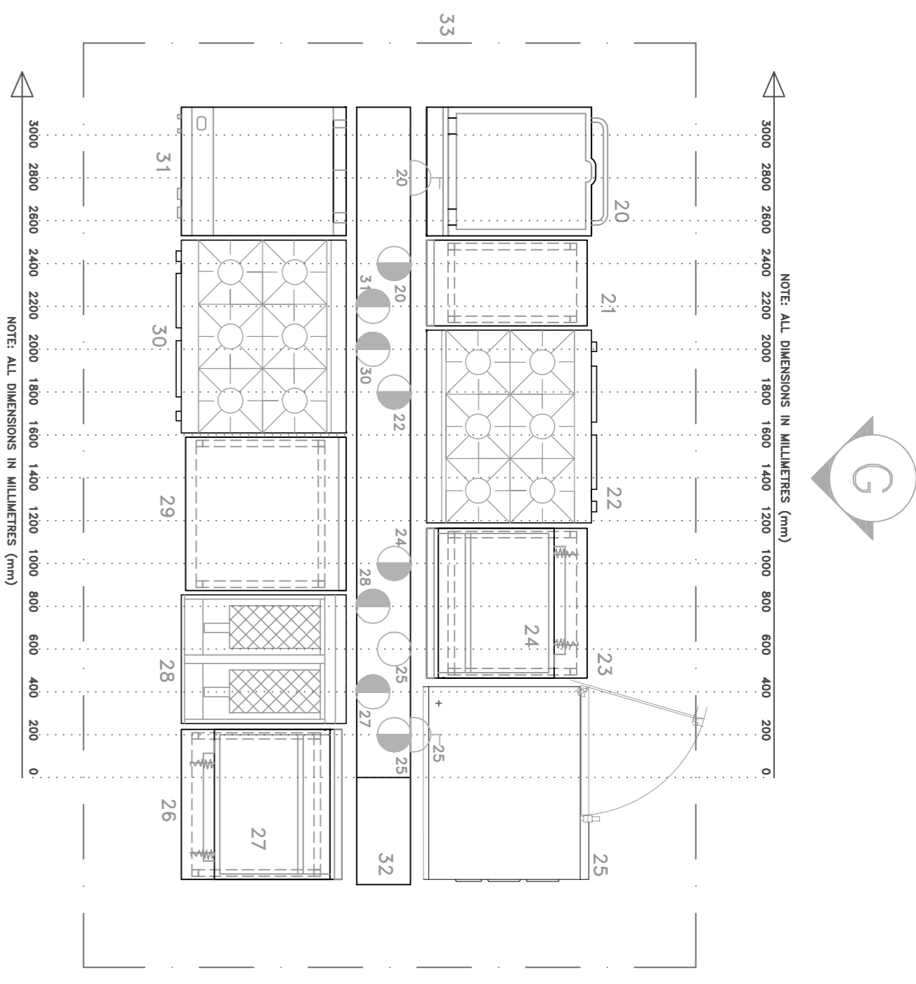
ELEVATION G
